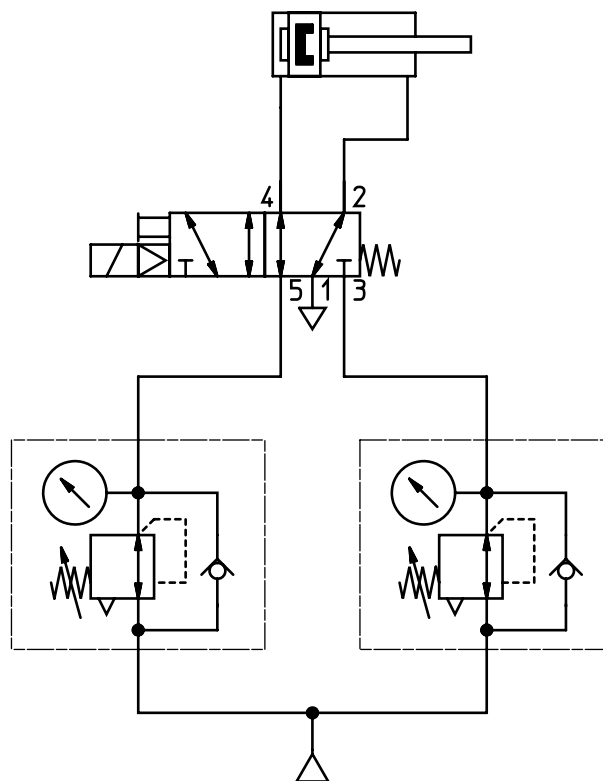
气路图 2: 调节阀上游的压力
