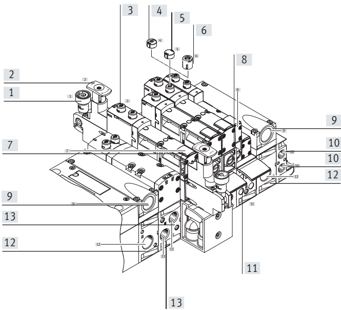
气接口和控制元件
