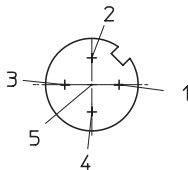
[1] 连接插头 M12x1, 5 针
