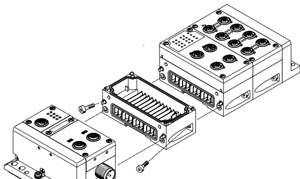
CPX 电气终端，金属型
