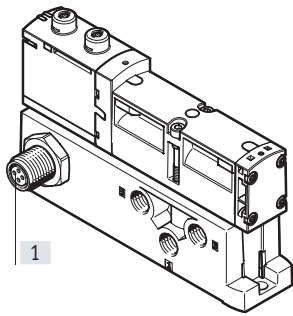
[1] 连接插头 M12x1, 4 针，符合 EN 61076-2-101
