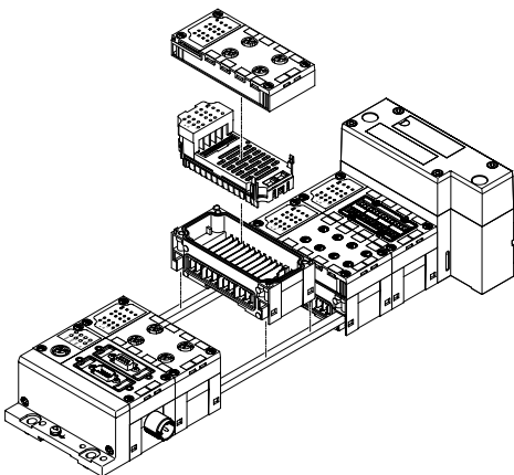
CPX 电气终端，金属型
