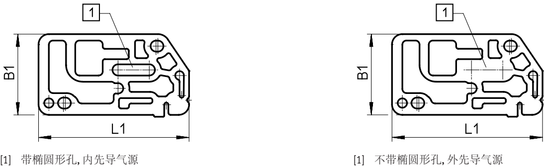
软启动阀和气路板之间的密封件 1)
