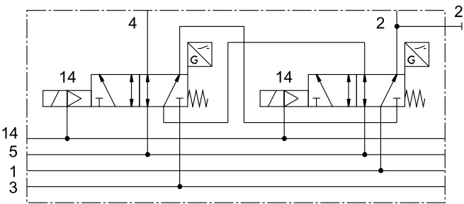
气路图 1)
