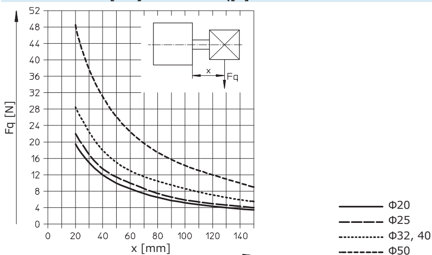
ワーク重心までの距離x[mm]時の許容横荷重Fq[N]
