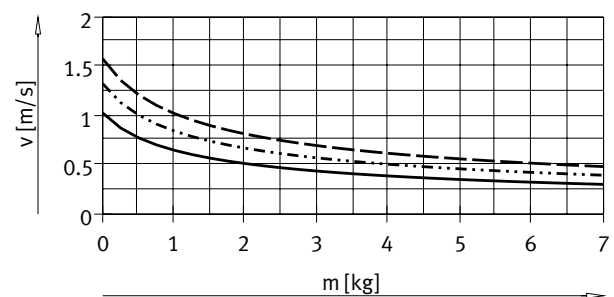
Piston \varnothing 20
