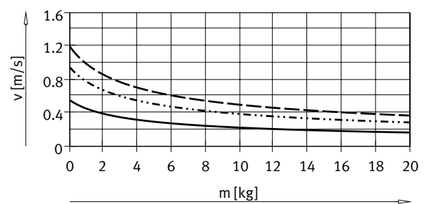
Piston \varnothing 32
