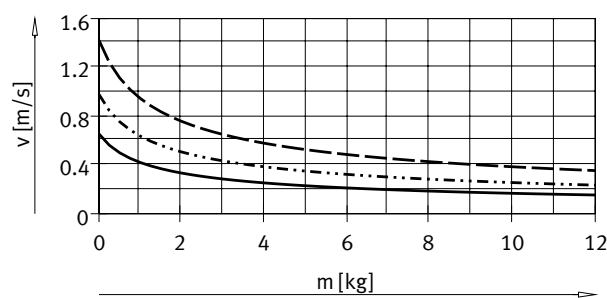
Piston \varnothing 25
