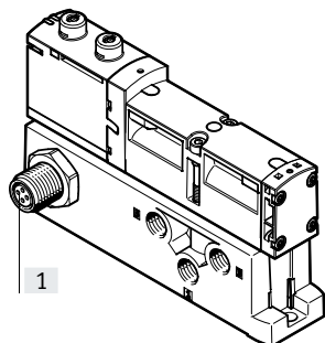
[1] Anschluss-Stecker M12x1, Stift, 4-polig nach EN 61076-2-101
