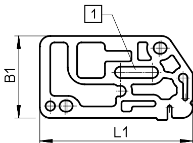
[1] mit Langloch, Steuerluftversorgung intern
