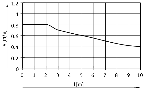
Für Baugröße 50
