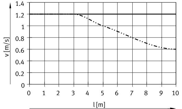
Für Baugröße 40
