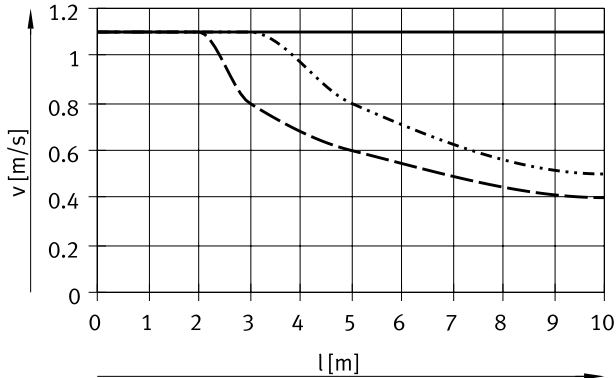
Für Baugröße 32
