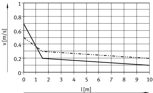
Für Baugröße 80
