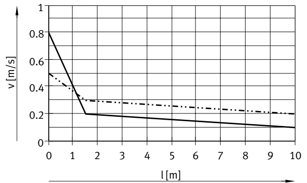
Für Baugröße 63
