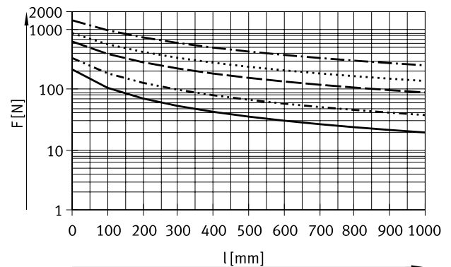
Querkraft senkrecht
