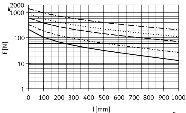
Querkraft waagrecht
