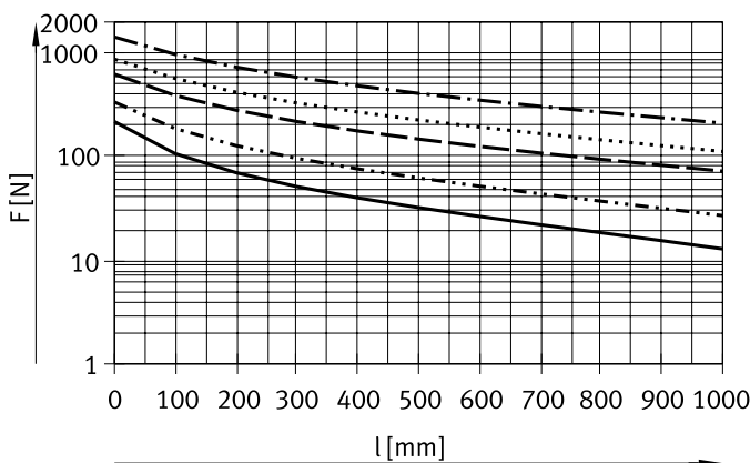
Querkraft waagrecht
