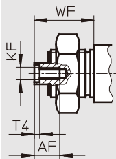
K3 - 피스톤 로드 암 나사산
