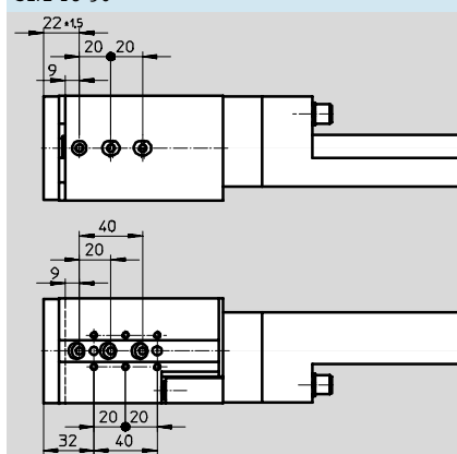
SLTE-16-50
