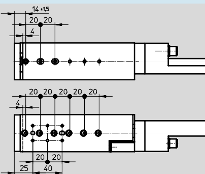
SLTE-10-80
