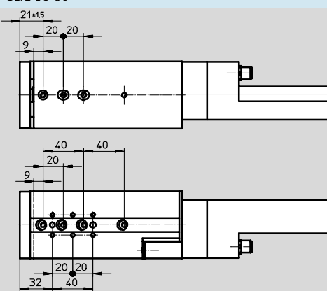
SLTE-16-80
