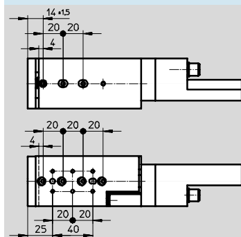
SLTE-10-50
