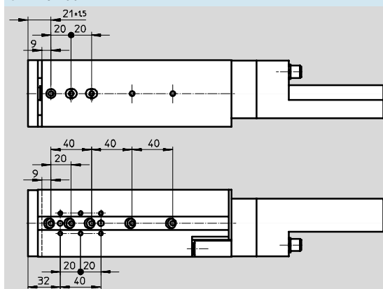
SLTE-16-100
