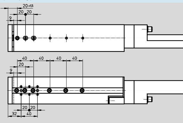
SLTE-16-150
