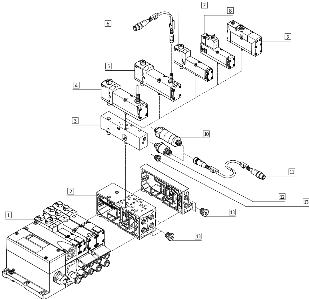
Cuadro general de periféricos - Válvula de conexión de pilotaje
