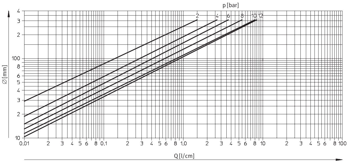
Luftverbrauch Q in Abhängigkeit vom Kolben-Ø und dem Betriebsdruck p
