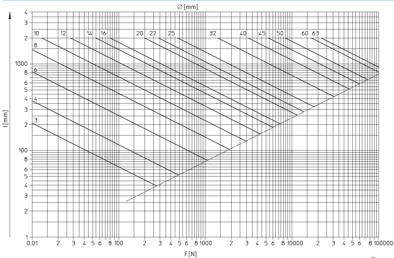
Kolbenstangen-Ø in Abhängigkeit von der Hublänge l und der Kraft F
