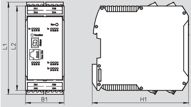
CMGA-B1-M2-L2-A0
