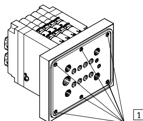
1 Otwory montażowe
