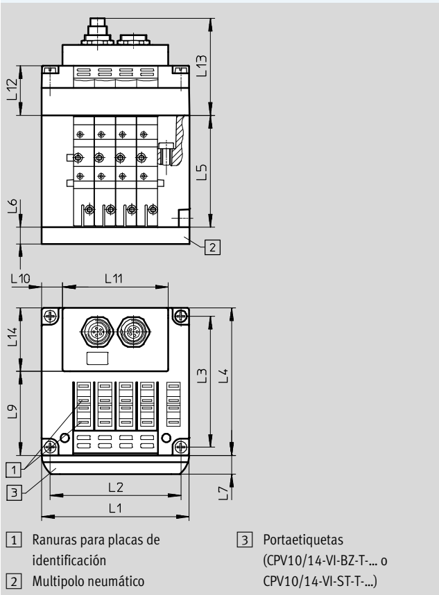
Terminal de válvulas con sistema de instalación CPI – CPV10/14
