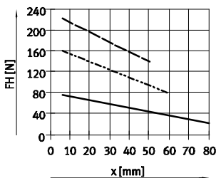
HGPT-50-A-F
