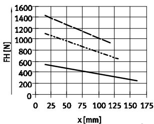
HGPT-50-A-F
