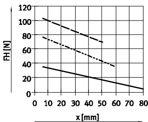
HGPT-50-A
