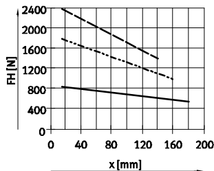
HGPT-63-A-F
