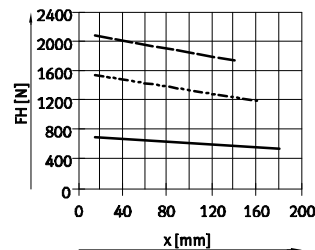
HGPT-80-A
