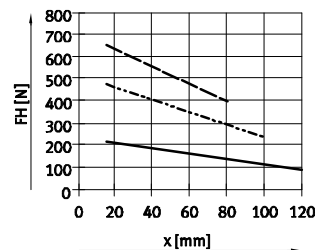
HGPT-80-A-F
