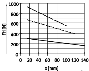
HGPT-40-A-F
