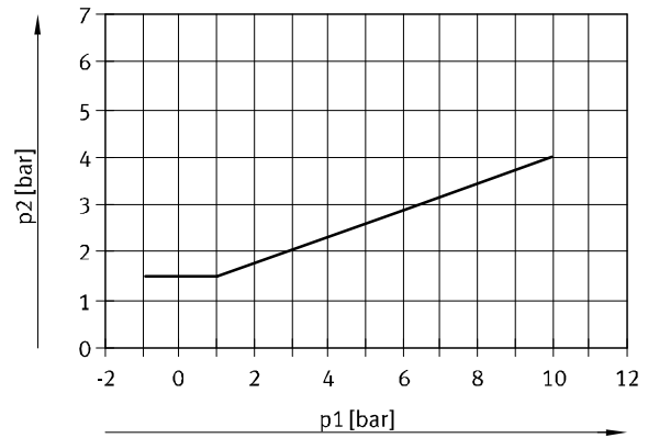
Steuerdruck p2 in Abhängigkeit vom Arbeitsdruck p1, Baugröße 25
