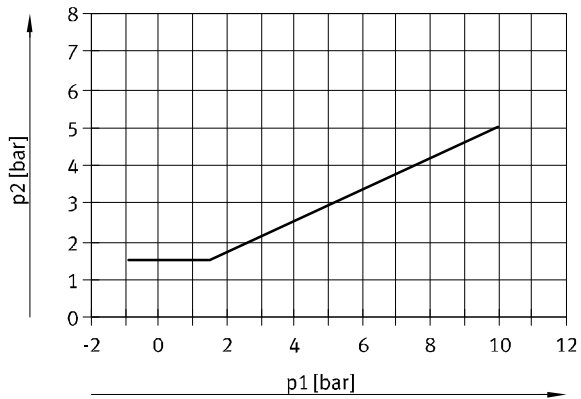
Steuerdruck p2 in Abhängigkeit vom Arbeitsdruck p1, Baugröße 20 für 3/2-Wegeventile
