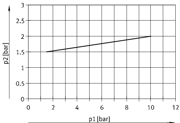
für 5/2-Wegeventile, bistabil
