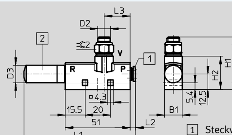
1 Steckverschraubung 2 Schalldämpfer
