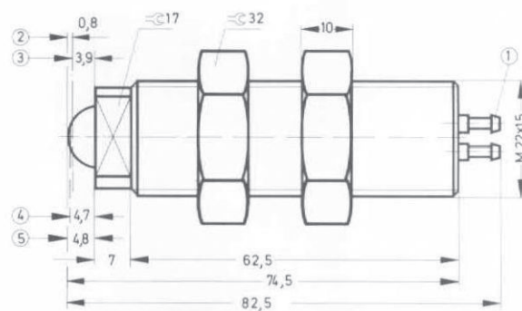
Typ SDK-4-PK-3
