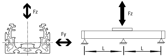
Kraft Fz
