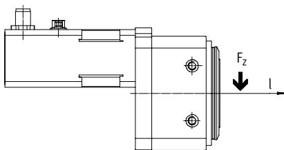
Max. dynamická radiálna sila F_z v závislosti na ramene páky l
