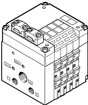
Terminal de válvulas AS-Interface con alimentación complementaria
