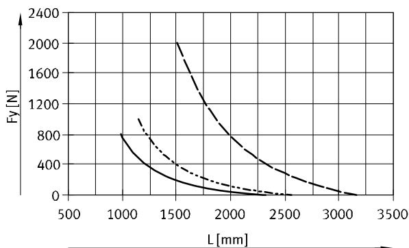
Fuerza Fy
