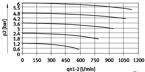
VPPM-6TA-...-0L6H-... (6 bar)
