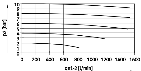
VPPM-6TA-...-0L10H-... (10 bar)
