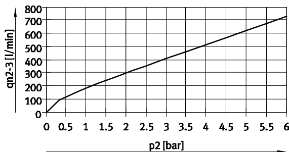
VPPM-6TA-...-0L6H-... (6 bar)
