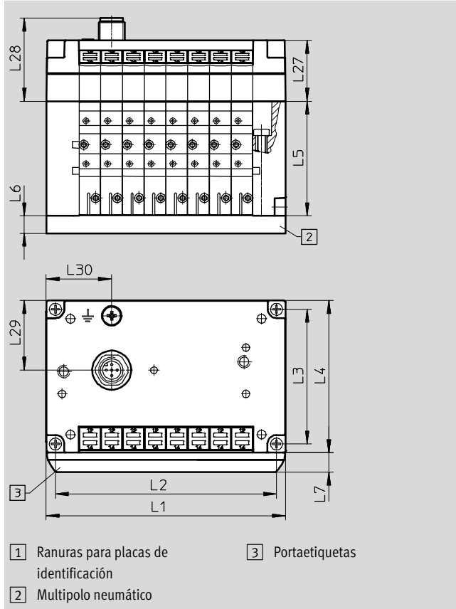
Terminal de válvulas con interfaz I-Port/IO-Link – CPV10/14
