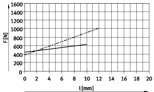
Tamaño 63 ... 80
