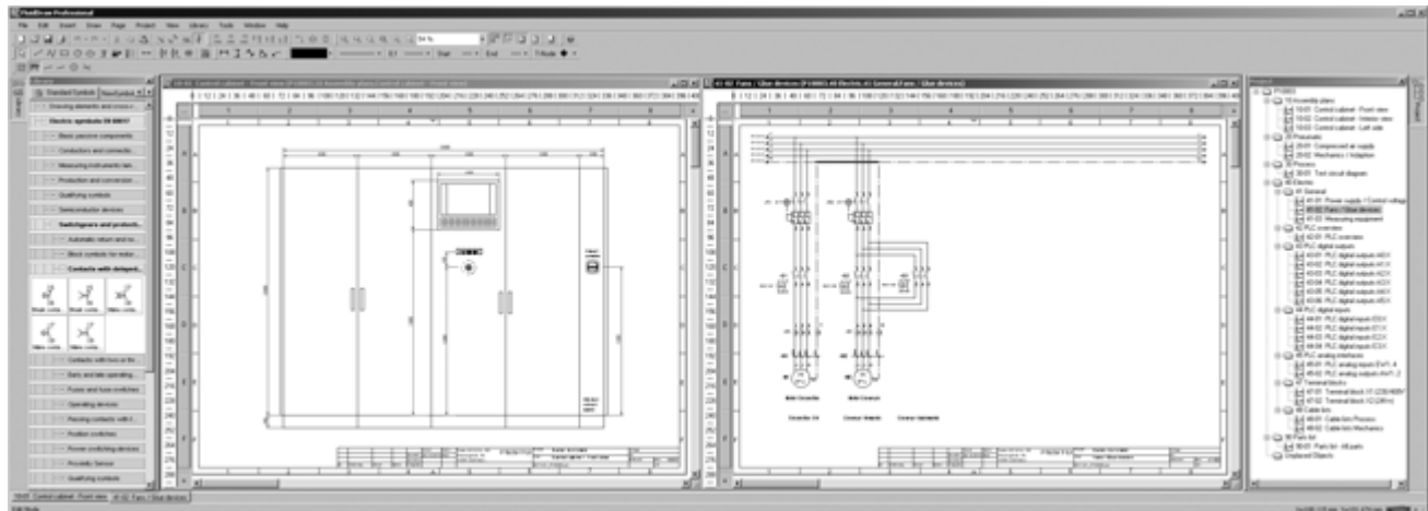
FluidDraw P5 con biblioteca de símbolos, esquemas de armarios de distribución, esquemas eléctricos y carpetas del proyecto.
