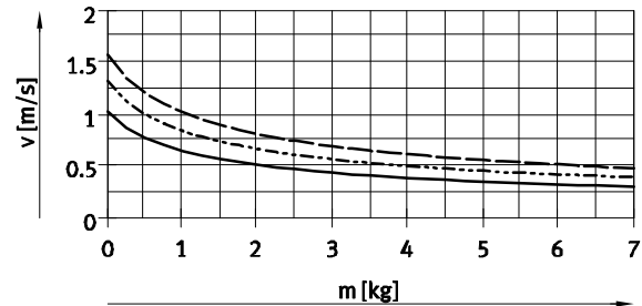
Diámetro del émbolo 20
