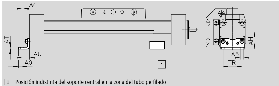
1 Posición indistinta del soporte central en la zona del tubo perfilado
