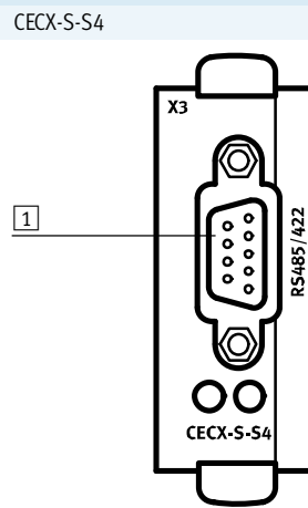
1 RS 485-A/422-A connection
