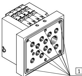
1 Montagebohrungen
