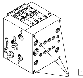
1 Montagebohrungen
