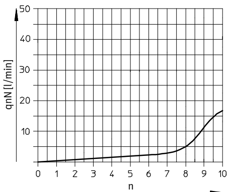
Normalnennendurchfluss q_{nN} bei 6 → 5 bar in Abhängigkeit der Spindelumdrehungen n
