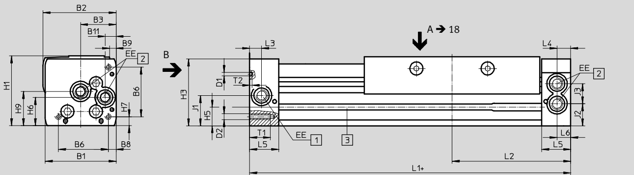
Ansicht B Ø 18
