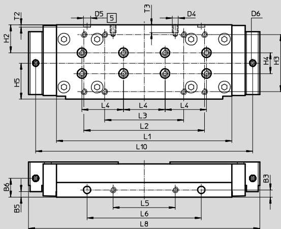
Ansicht A
