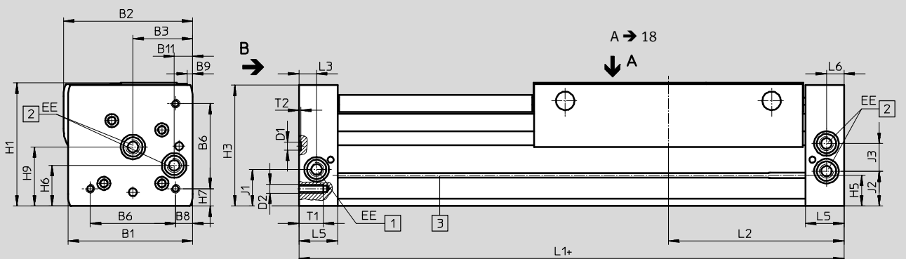
Ansicht B
