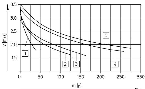
最大许用冲击速度 v 与应用负载 m 的关系
