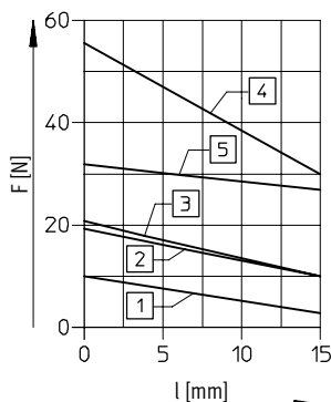
最小弹簧复位力 F 与行程 l 的关系
