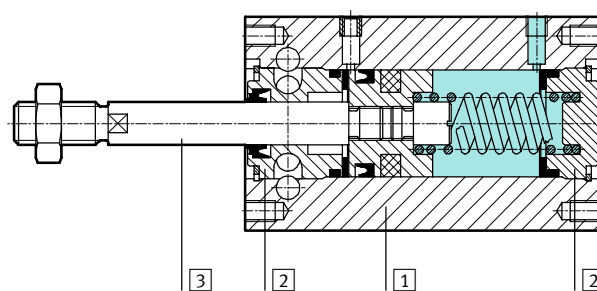
剖面图 EMM(L)Z - 拉
