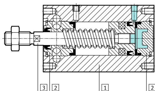
剖面图 EMM(L) - 推
