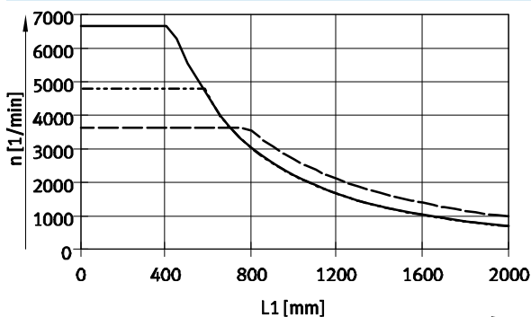
Número de revoluciones n máximas en función de la distancia nominal L1
