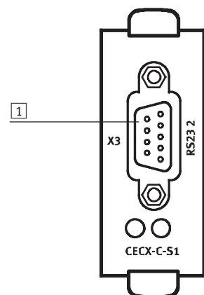
1 Conexión RS 232
