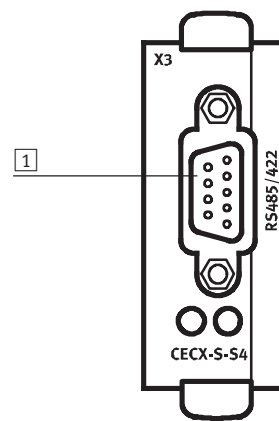
1 Conexión RS 485-A/422-A
