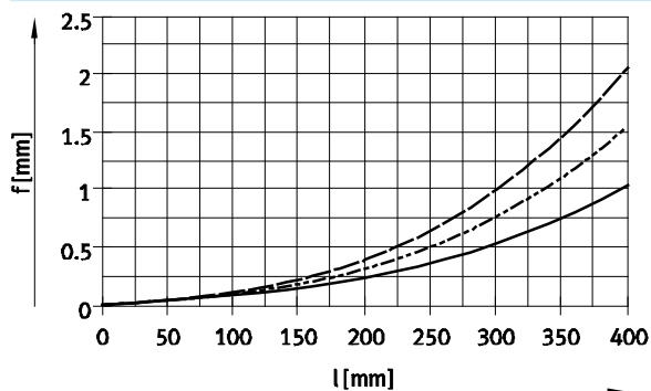
DFME-40
