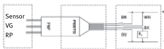
Kabelbaum zur VADMI Verzweigung SPS (kundenseitig)
