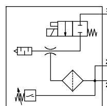
VADM-...-P/-N mit Vakuumschalter
