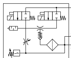
VADMI-...-P/-N mit Abwurfimpuls und Vakuumschalter
