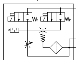
VADMI-...-P/-N mit Abwurfimpuls und Vakuumschalter
