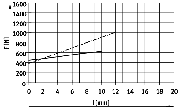
Baugröße 63 ... 80
