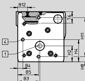
Ansicht B
