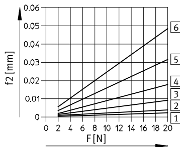
Kolben-Ø 10 mm
