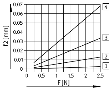
Kolben-Ø 4 mm
