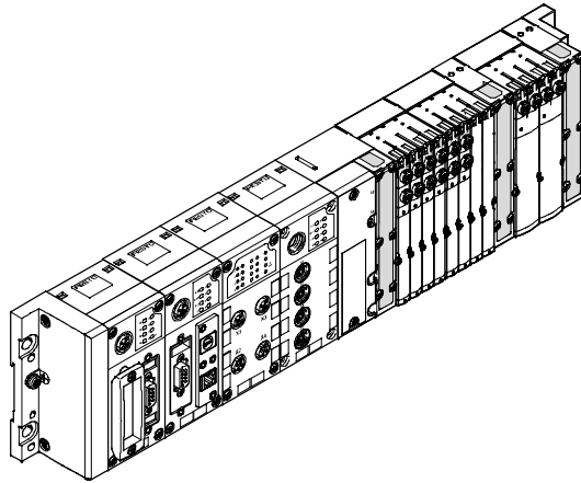
Esecuzione in metallo con unità di valvole VTSA - centrale
