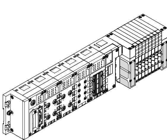
Con unità di valvole CPA - centrale
