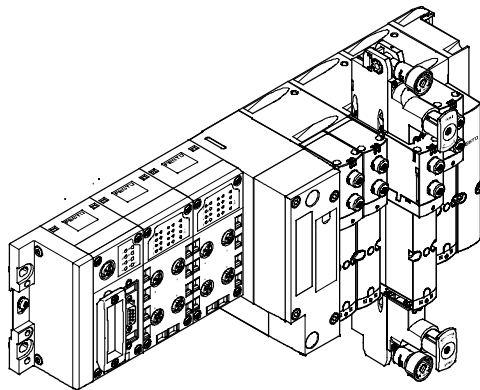
Con unità di valvole MIDI/MAXI - centrale
