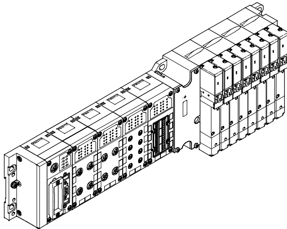
Con unità di valvole MIDI/MAXI - centrale
