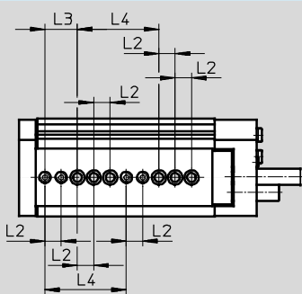
DGSL-12-50 ... 100
