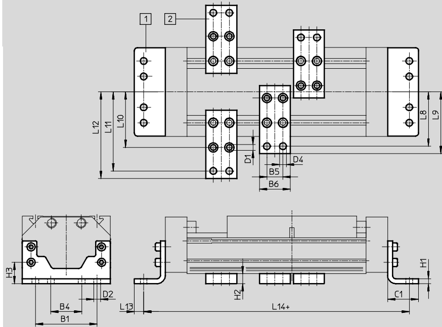
DGE...-HD18/-HD25/-HD40
