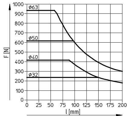
Carrera 250 ...400 mm
