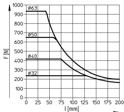
Carrera 200 ...400 mm
