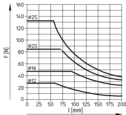
Carrera 125 ...200 mm
