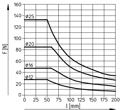
Carrera 40 ...100 mm
