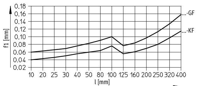
DFM con 2 apoyos por barra de guía
