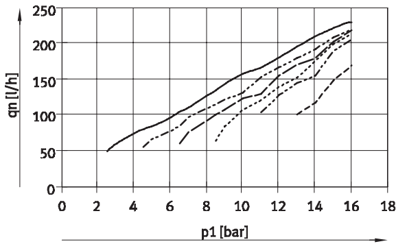
LFR/LFRS-...-MAXI
