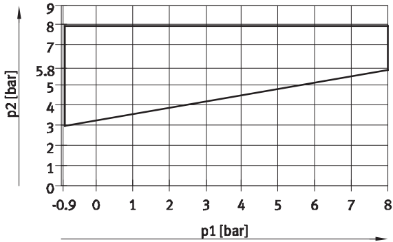
Presión de pilotaje p_2 en función de la presión de funcionamiento p_1 para válvulas con reposición por muelle mecánico (MPA1) para válvulas con código NS, KS, HS, DS
