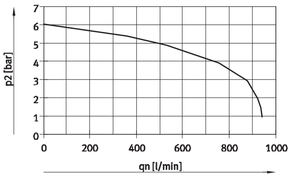
Caudal q_n en función de la presión de salida p_2 con placas reguladoras de presión (placas B), para conexión 2 Ancho de 21 mm
