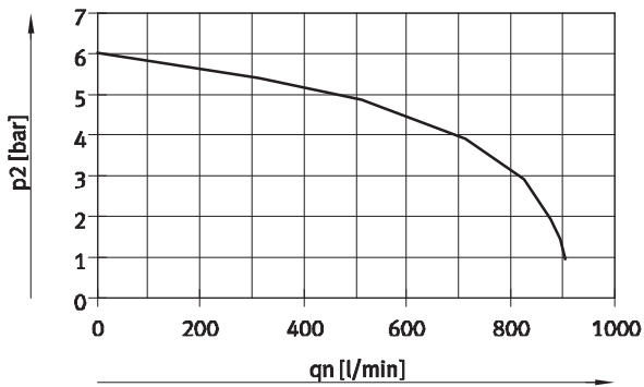
Caudal q_n en función de la presión de salida p_2 con placas reguladoras de presión (placas P), para conexión 1 Ancho de 21 mm
