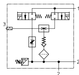
VADMI-...-P/-N 带喷射脉冲和真空开关
