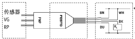
线束, 连接 VADMI
