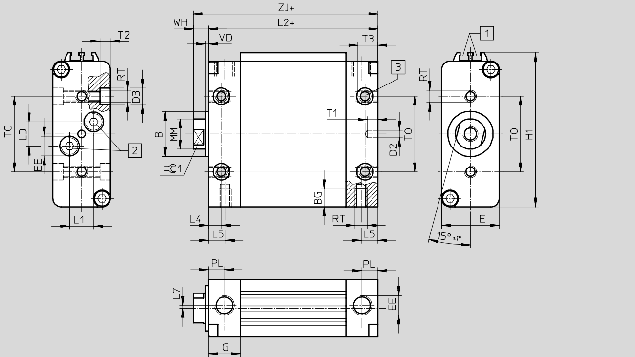
① 接近开关安装槽 ② 附加气接口, 用堵头密封 ③ 最大紧固扭矩 + = 加工作行程
