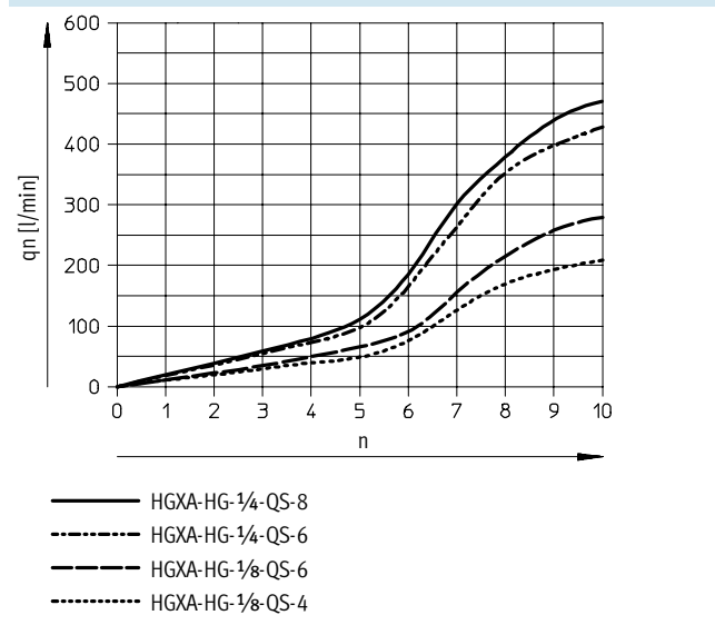
Portata normale qn a 6 bar → 0 bar in funzione del numero di giri della vite n Regolatore di portata unidirezionale
