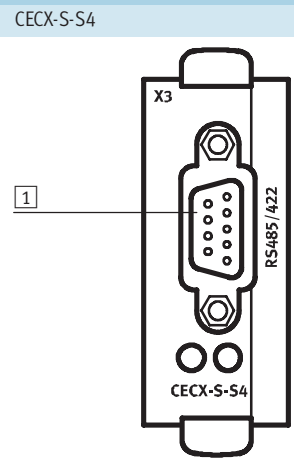
1 RS 485-A/422-A connection
