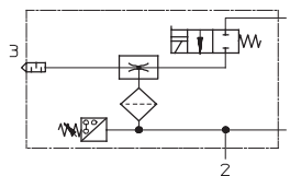
VADM-...-P/-N mit Vakuumschalter
