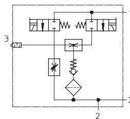
VADMI-...-P/-N mit Abwurfimpuls und Vakuumschalter
