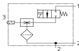
VADM-...-P/-N mit Vakuumschalter
